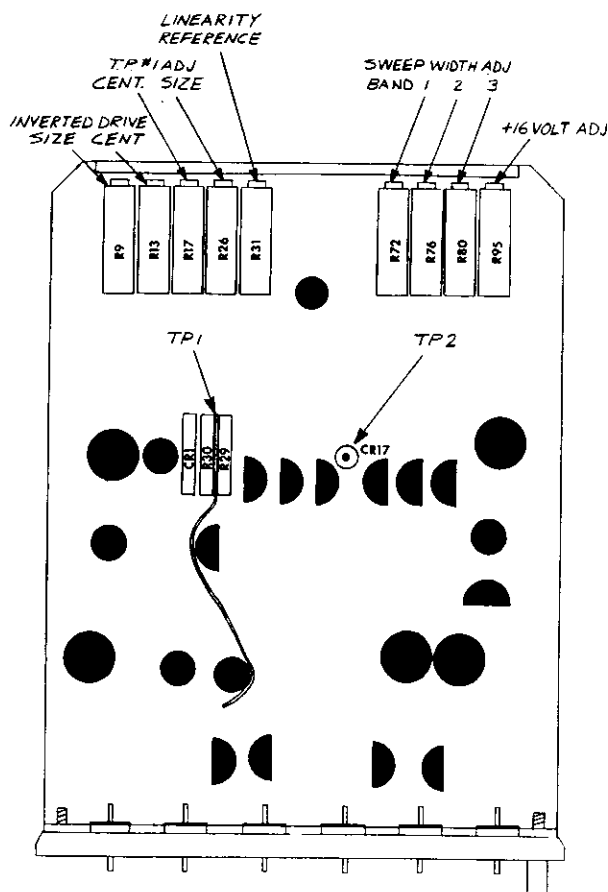
Figure 5-9. M2H Module
